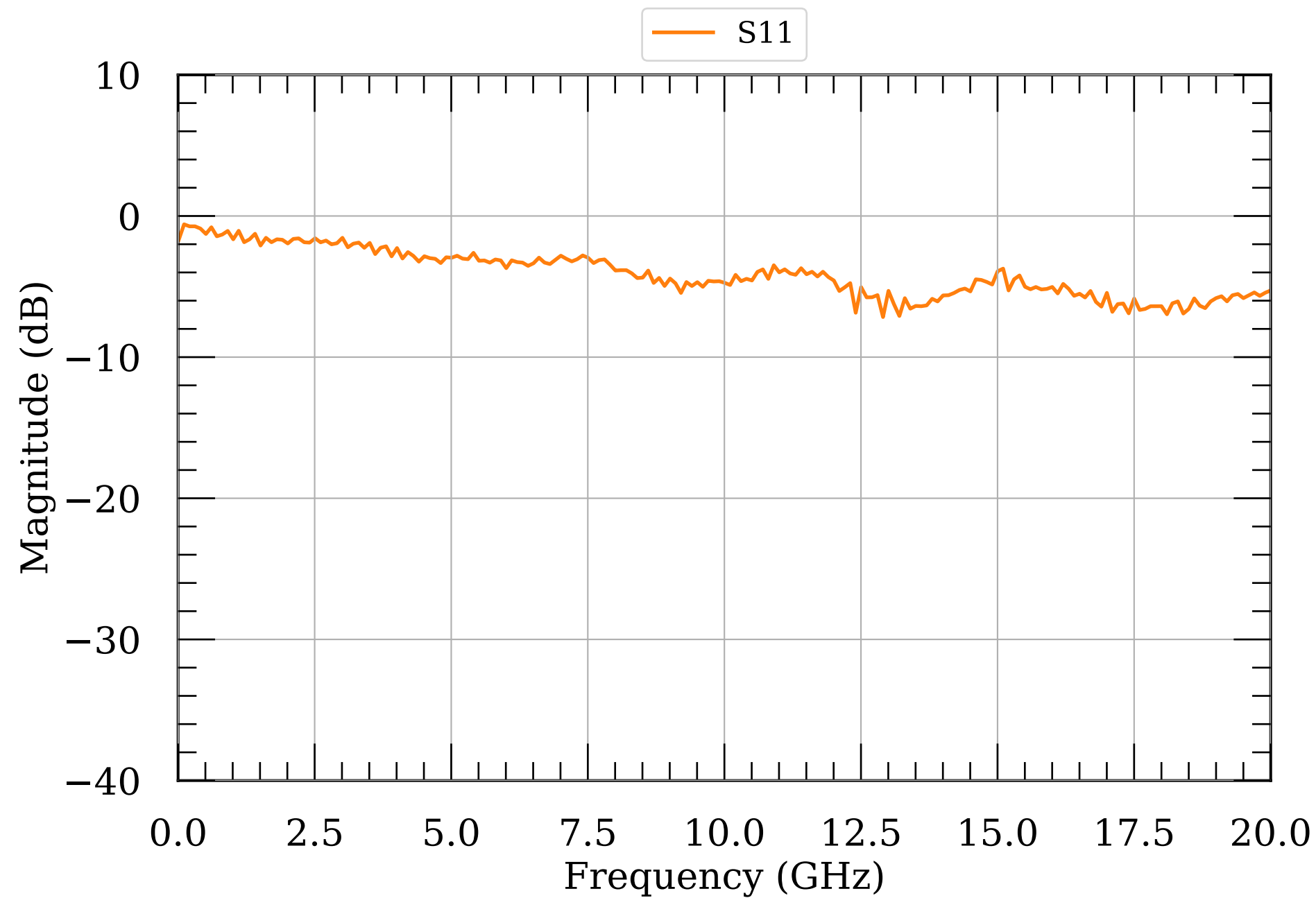
LNA S-params module037
